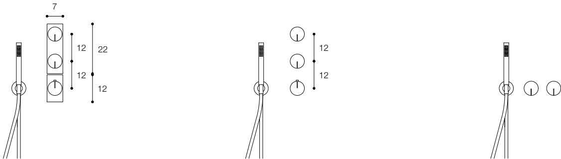
Gruppo doccia / Shower set
