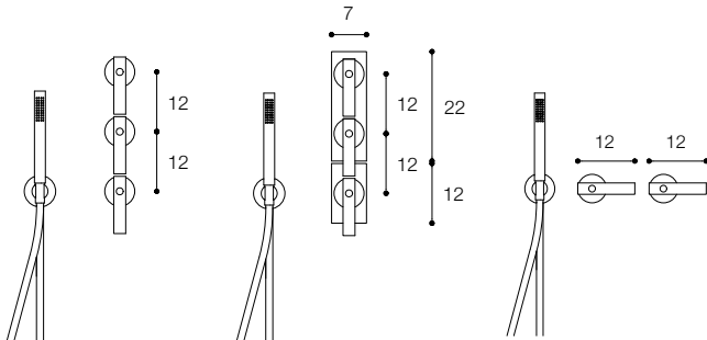
Gruppo doccia / Shower set
