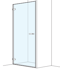
Pendeltüre Wandanschlag in Nische
