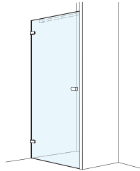
Flügeltüre Wandanschlag in Nische
