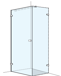
Flügeltüre Wandanschlag mit Seitenwand
