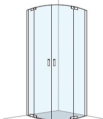
Viertelkreisdusche mit Pendelement und Festelementen
