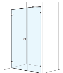
Flügeltüre Wandanschlag mit Seitenwand in Flucht
