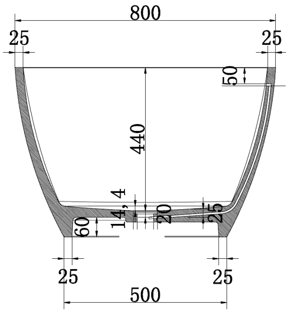
Querschnitt
