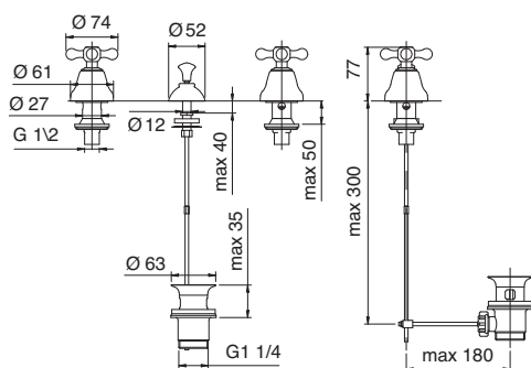
3620 Batteria bidet senza canna 3 hole bidet without spout (D RTVT101)
