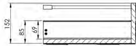
Tiroir avec railings - Vue profil
