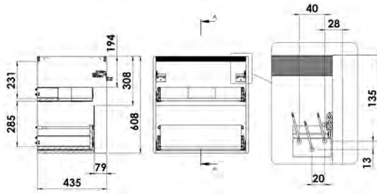
Tiroir simple - Vue profil
