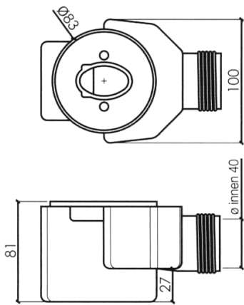
Ablauf H = 81 mm für die Rinne
